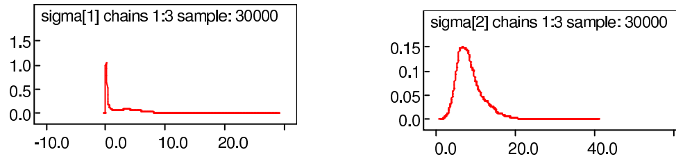
(b) Posterior densities of variances
