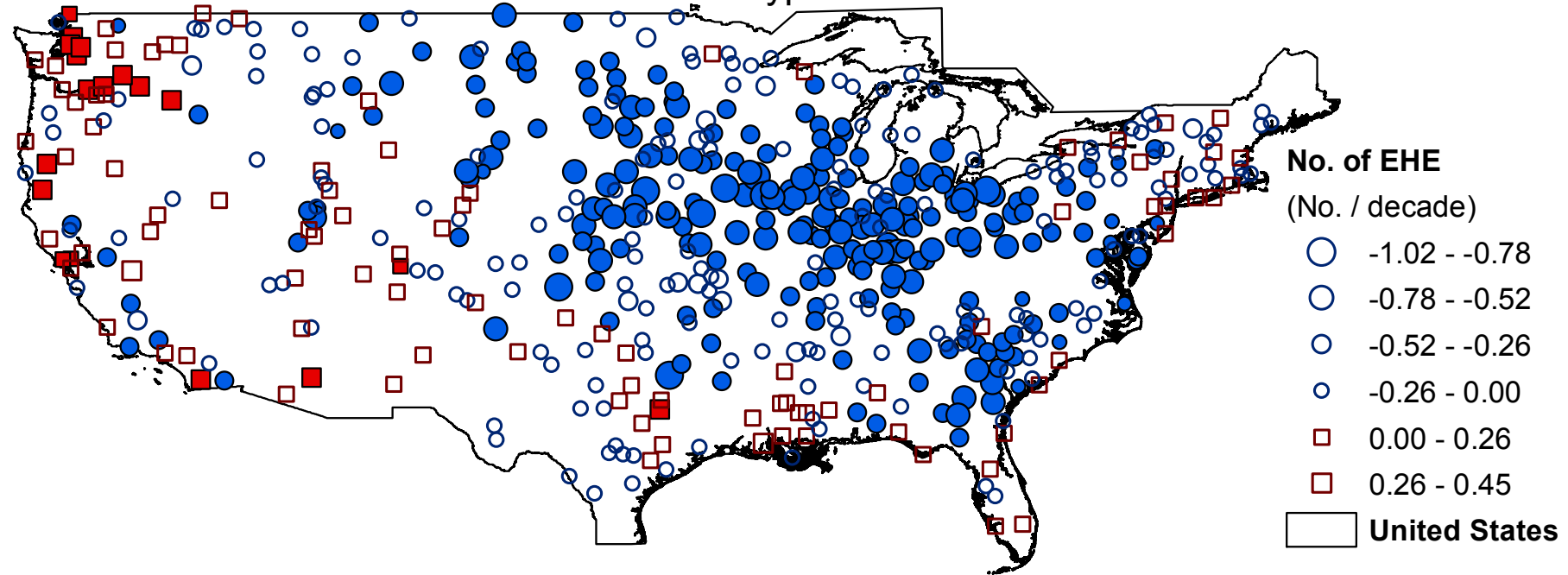
Tmin&max type EHE trends from 1930-1970
