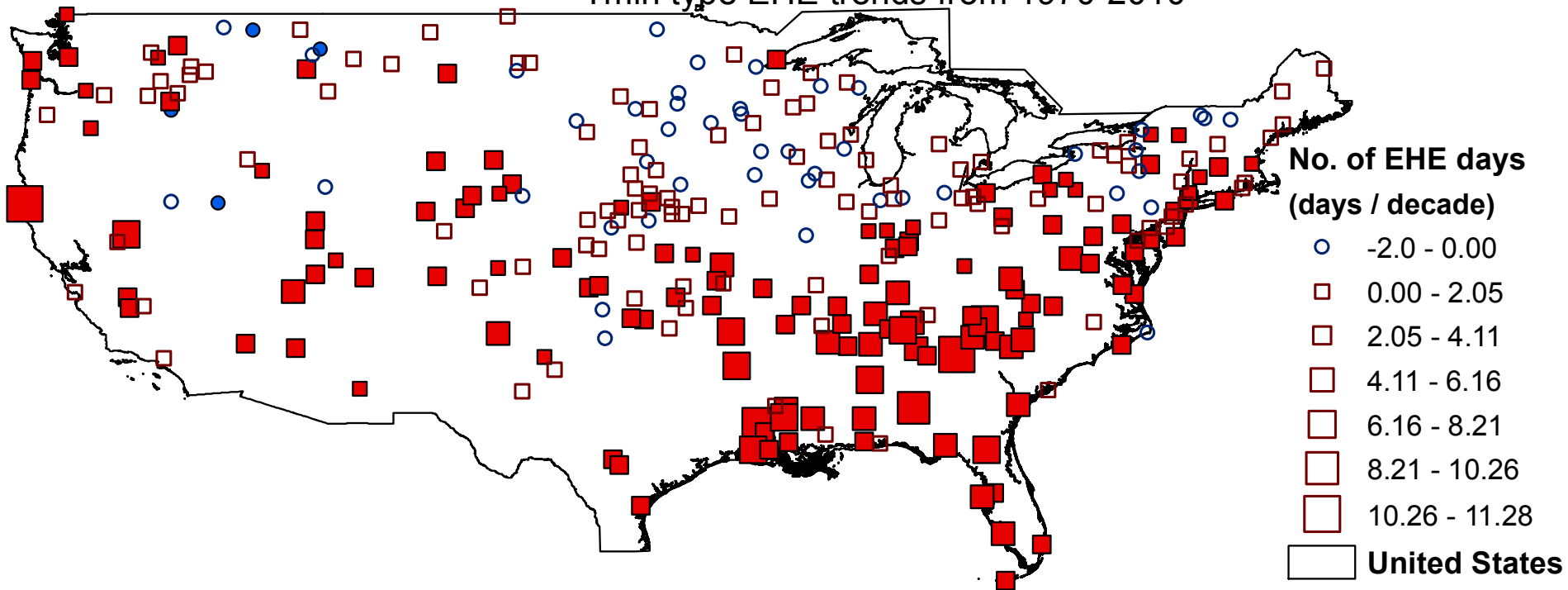
Tmin type EHE trends from 1970-2010
